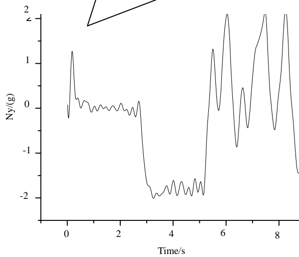
图1 飞行试验记录的过载曲线
